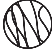
Pluto
