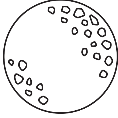
Uranus
